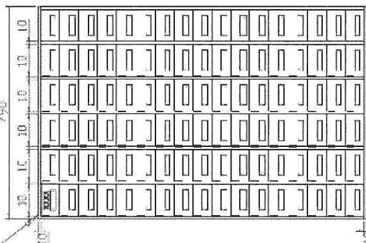
102格手機櫃(D280mm)
